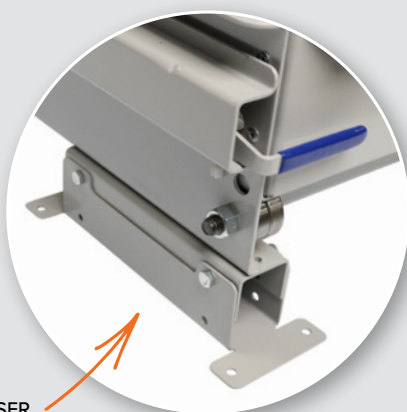
RISER BRACKET
