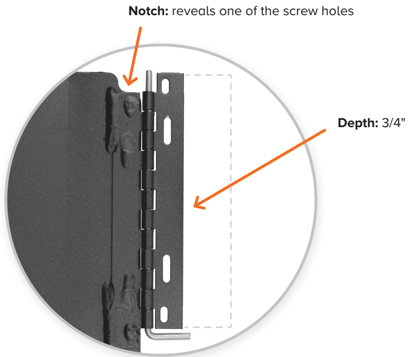
HINGE 2
